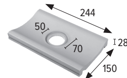
Canaleta con desagüe Drainage overflow channel
