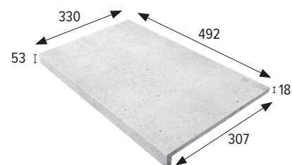
Peldaño recto 50 · Straight stair-tread 50
