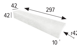
Cantonera transición Ext. radial transition tile
