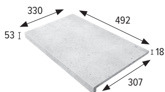
Peldaño recto 50 Straight stair-tread 50
