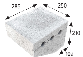
Pieza nicho B-33 B-33 Niche piece
