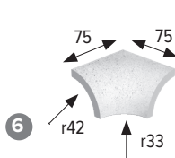
Esq. int. rinconera Internal mitre
