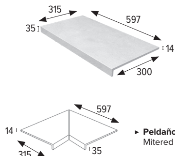
Peldaño recto 60 · Straight stair-tread 60
