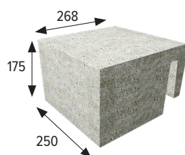
Pieza maciza esquina de nicho/ancraje corchera Niche corner piece/lane rope fixing piece
