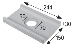
Canal con desagüe Duct
