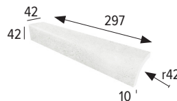
Cantonera transición Ext. radial transition tile
