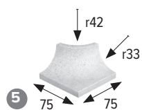
Esq. ext. cantonera External mitre
