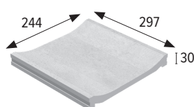
Canaleta · Overflow channel*
