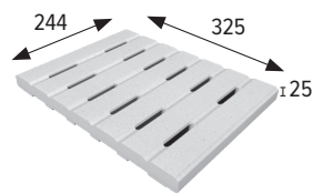
Rejilla cerámica monocompact Monocompact ceramic grid **
