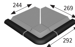
Esq. ext. borde GA SPA GA SPA edge ext. corner
