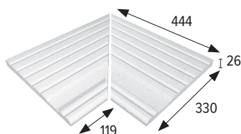
Rejilla cerámica monocompact Monocompact ceramic grid **
