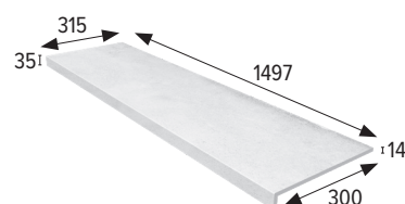
Peldaño recto 180* · Straight stair-tread 180 * Disponible bajo pedido. / Available on demand.
