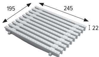
Rejilla long. rígida 195 mm Grating 195 mm - Rigid longitudinal
